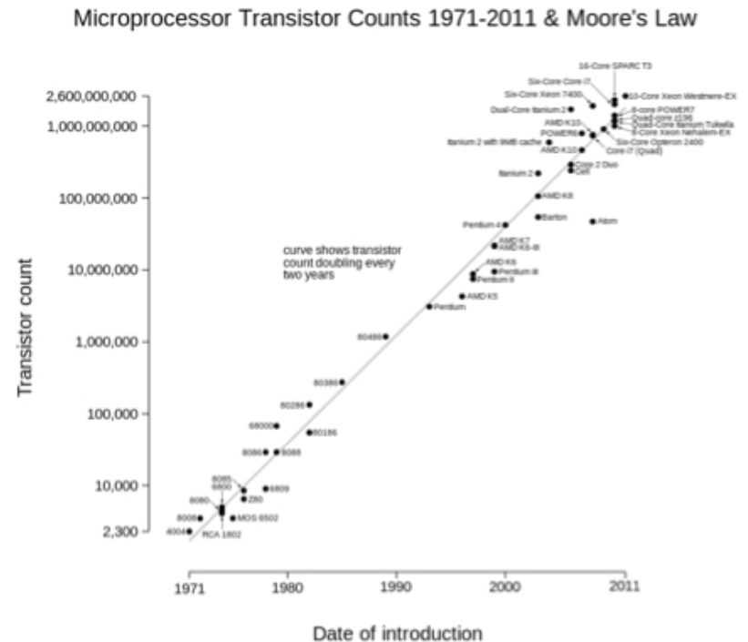
Figura 1.4 Ley de Moore
